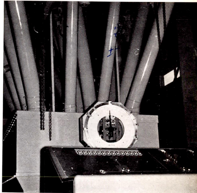
パンチカード コントロール デスク 26 工場の心臓部に当り、原料から製品まで自動制御します
