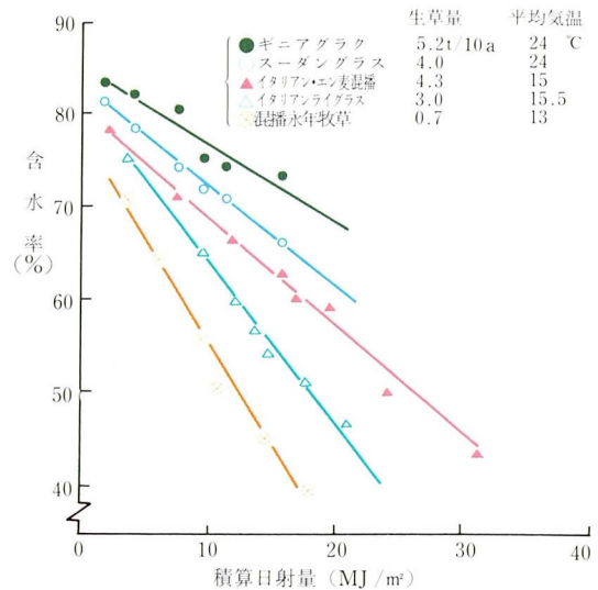
図2 牧草の圃場乾燥速度（1日2～3回転草） 空きやすい。
