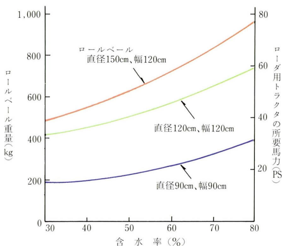
図3 ロールベールの水分と重量の関係 (定径型ロールベール)
