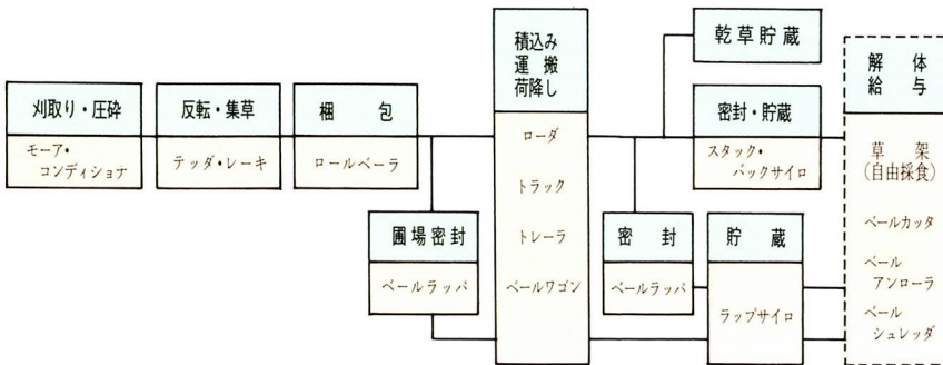
図1 ロールベールサイレージ収穫作業体系
